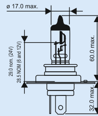
H4
