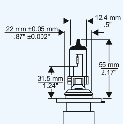
9006XS
