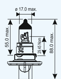
H13/9008
