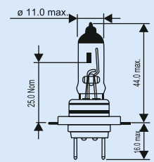
H7
