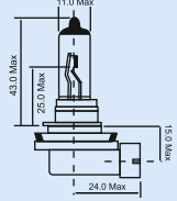
H11
