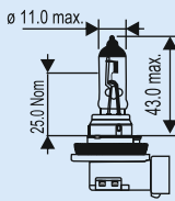
H8
